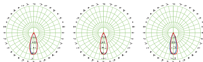
配光角度
