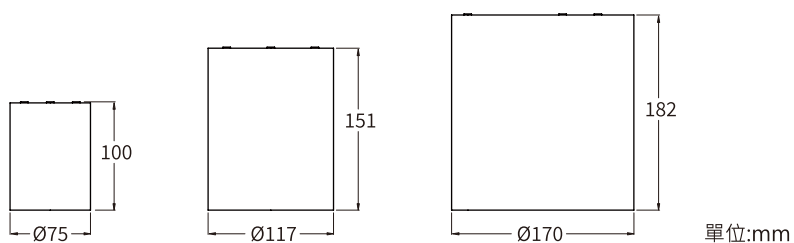
產品尺寸
