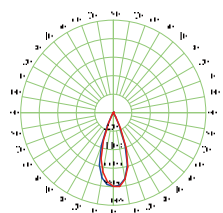
配光角度
