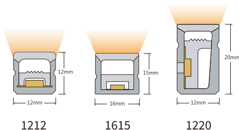
產品尺寸
