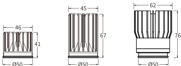
產品尺寸
