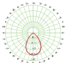
配光角度
