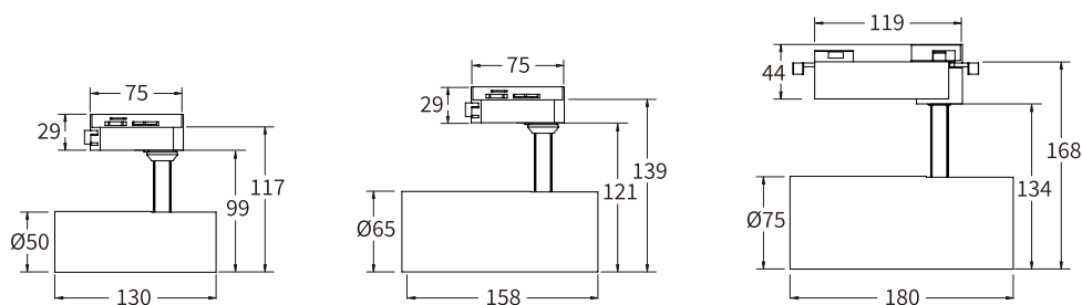
產品尺寸
